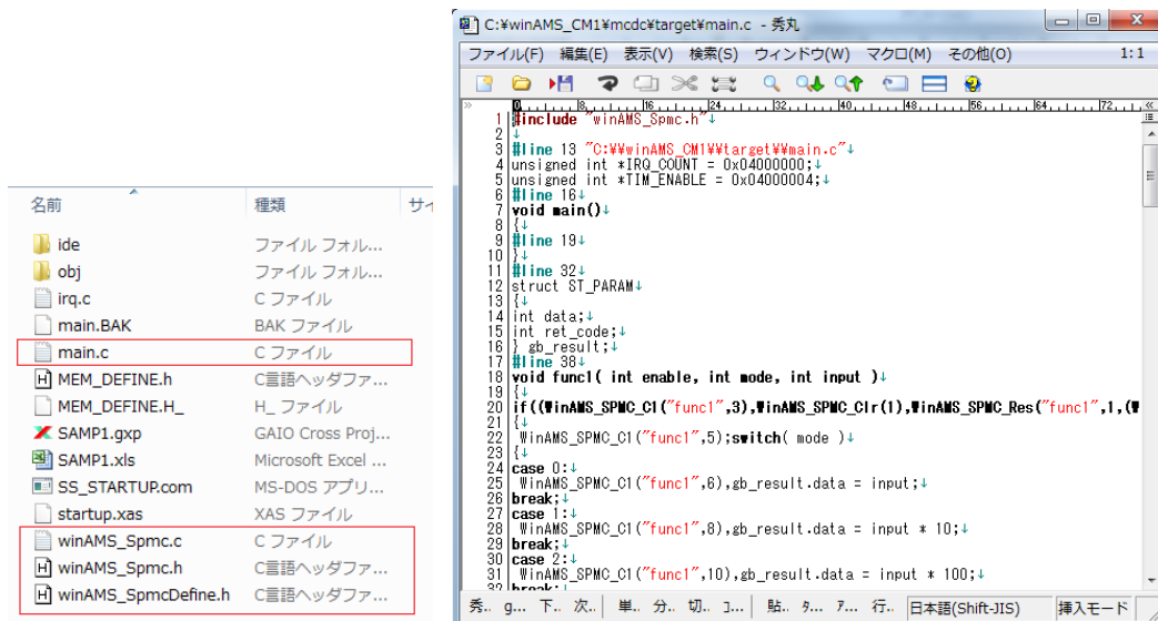
フック関数の本体を含むソースファイル(winAMS_Spmc.c)と フックコードが挿入された main.c
